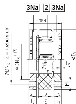
wykonanie DFN
